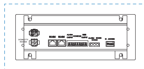
圖C 控制器面板
