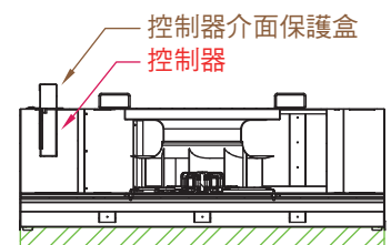
剖面圖 B-B
