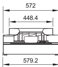
剖面圖 B1-B2
