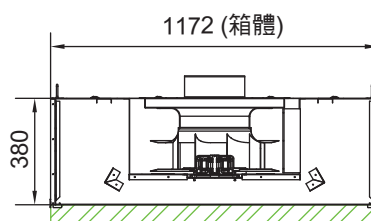
剖面圖 A-A
