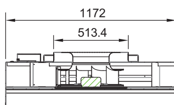
剖面圖 B-B
