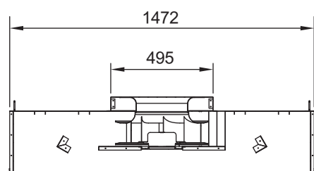
剖面圖 A1-A2
