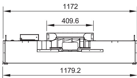
剖面圖 A1-A2
