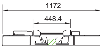
剖面圖 A-A
