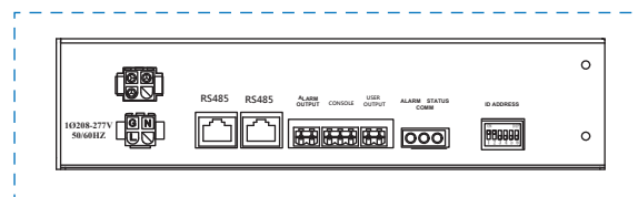
控制器面板
