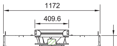
剖面圖 B-B
