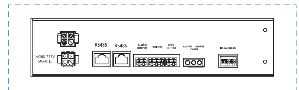
控制器面板(4:1)
