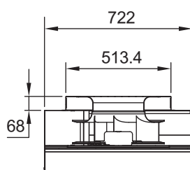
剖面圖 B1-B2
