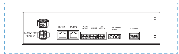
控制器面板
